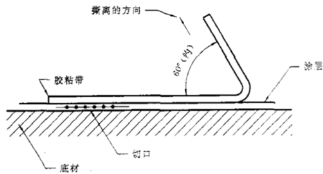
a) 根据网格定胶粘带的位置
