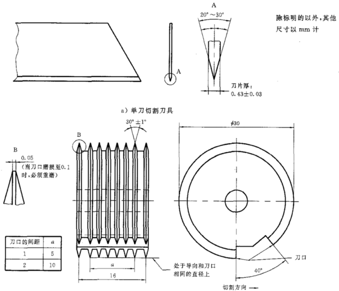
图 1 适合的切割刀具
