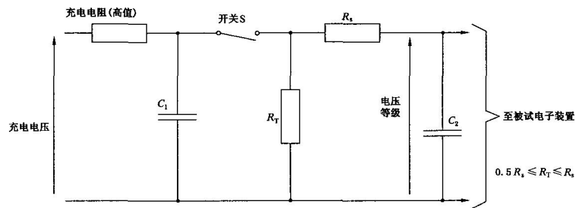
a) 试验电路
