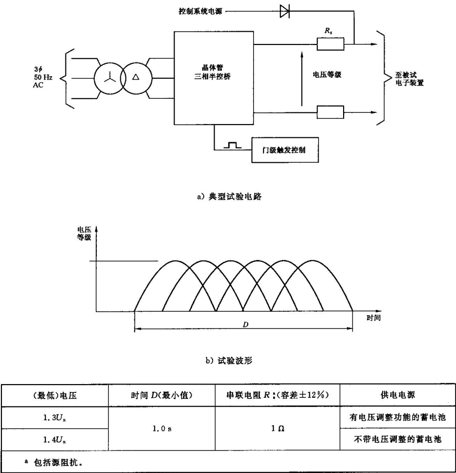
图 3 可采用的电源过电压试验
