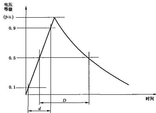
b) 试验波形
