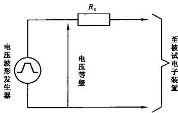
a) 试验电路
